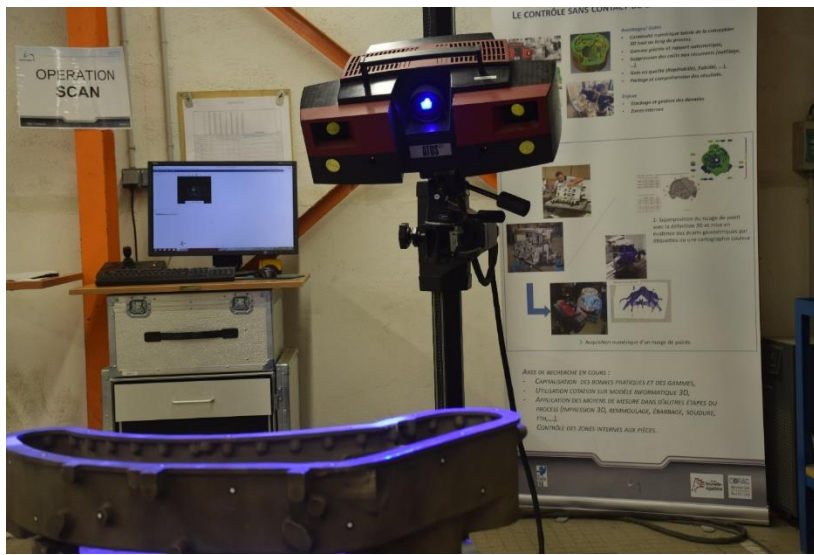
Contrôle géométrique sans contact pièce Ventana Arudy
